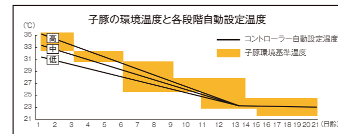
ワンタッチBOXは日齢に応じた子豚にとって快適な温度が保てます
